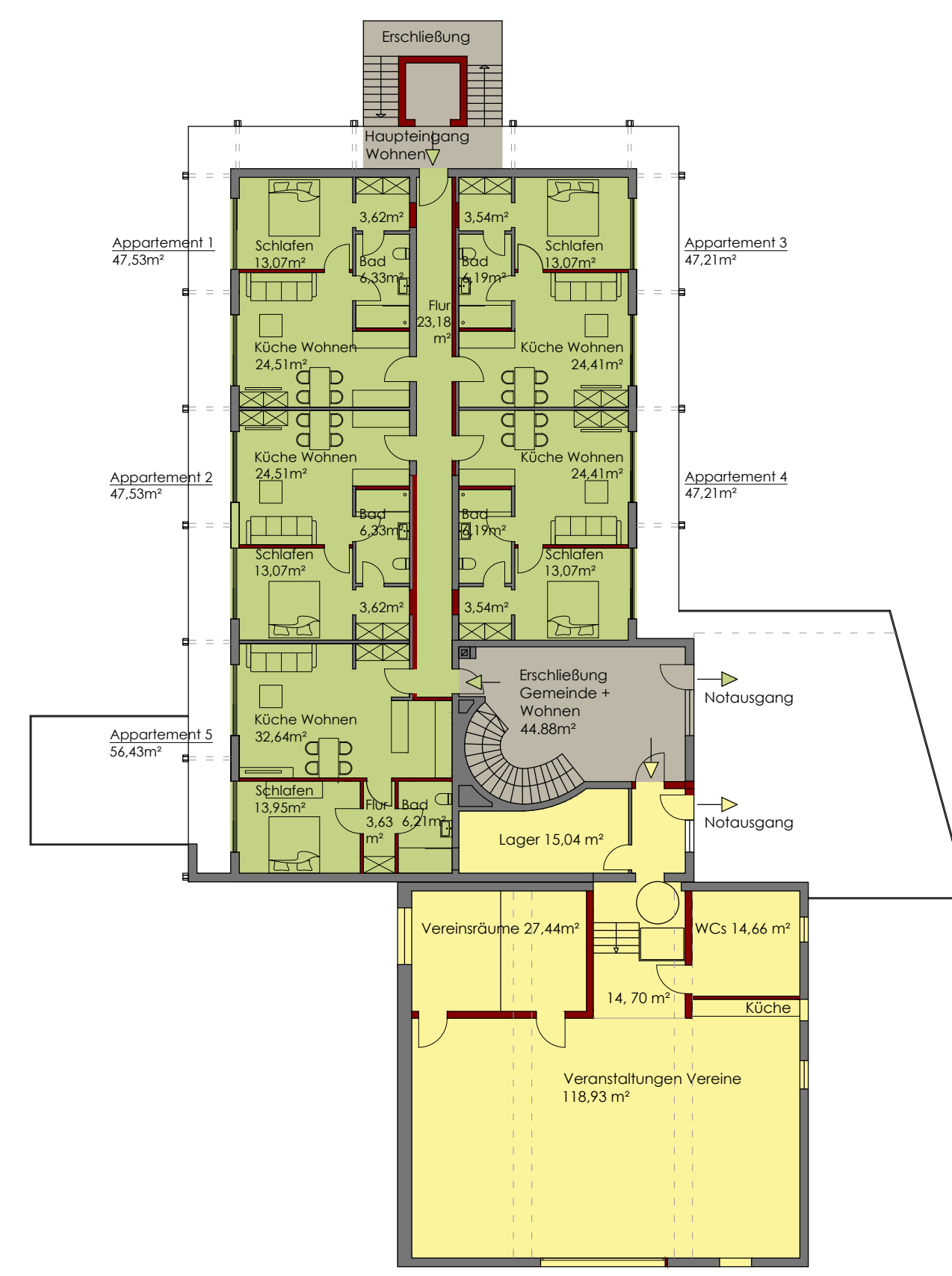
VARIANTE 2 Grundriss OG 1-200 Gemeinde + 5 Apartments
