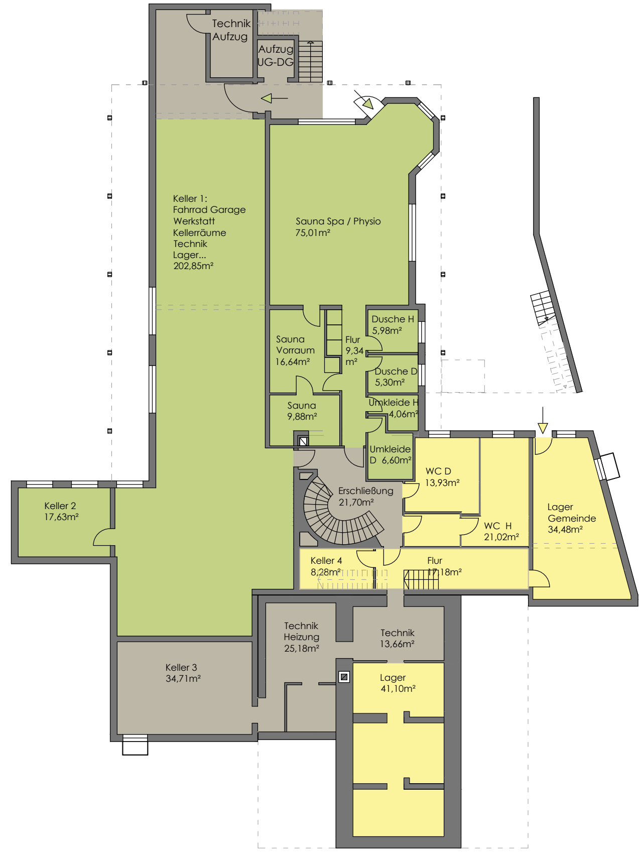
VARIANTE 2 Grundriss UG 1-200 Technik, Kellerräume, Toiletten
