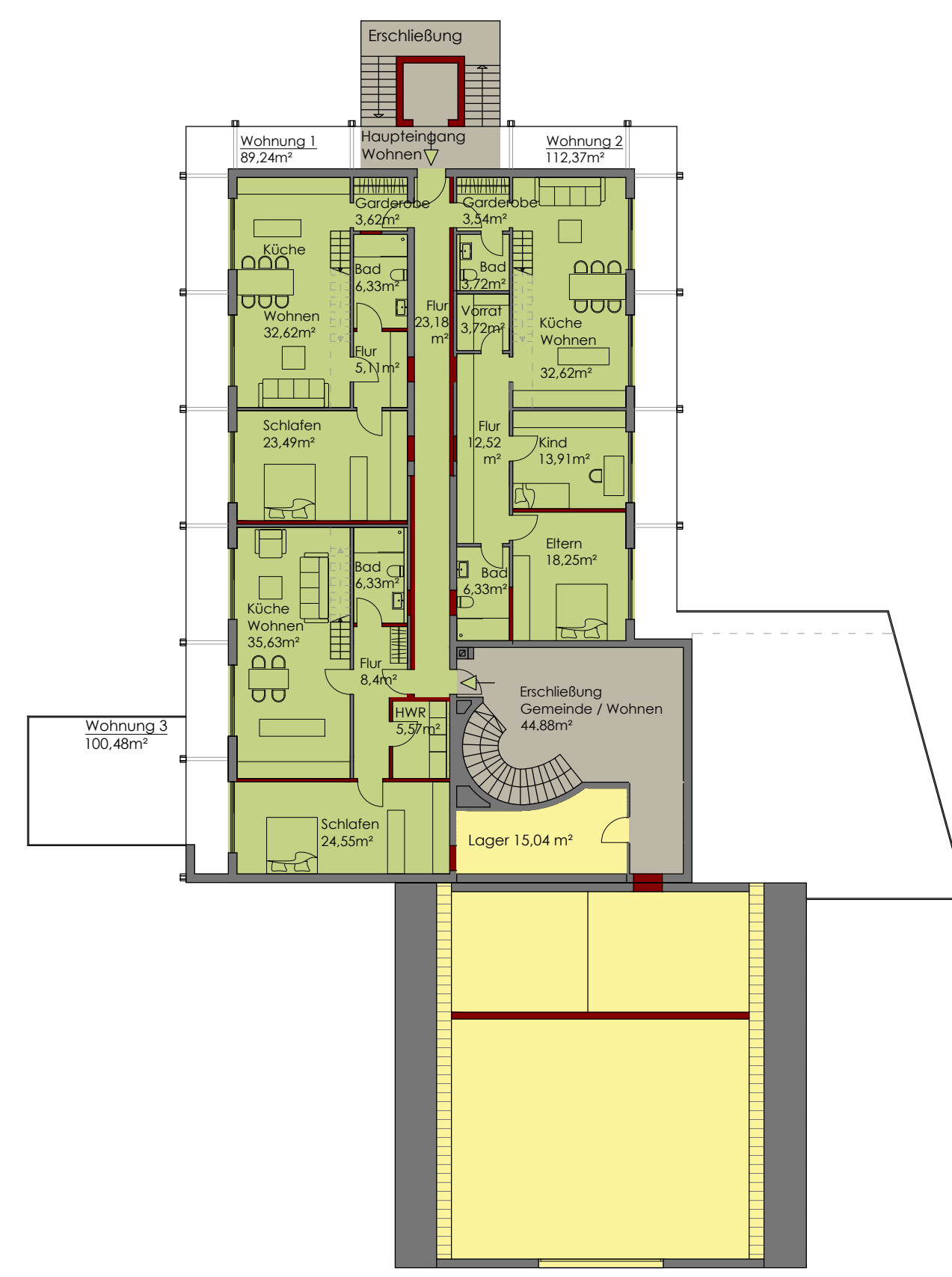
VARIANTE 2 Grundriss DG 1-200 3 Wohnungen
